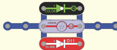
Paralelní obvod
