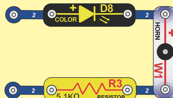
Sériový obvod
