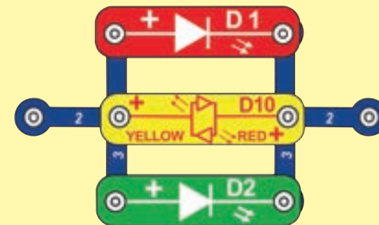
obwód równoległy
