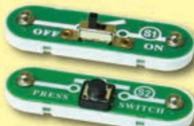
Przełącznik suwakowy i przycisowy (S1 i S2)
