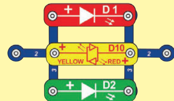
Paralelní obvod
