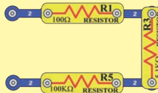
Obwód szeregowy
