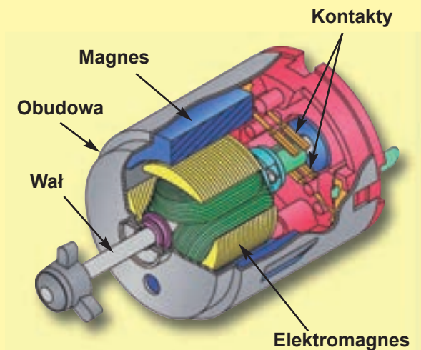
Silnik (M1)
