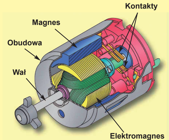
Silnik (M1)
