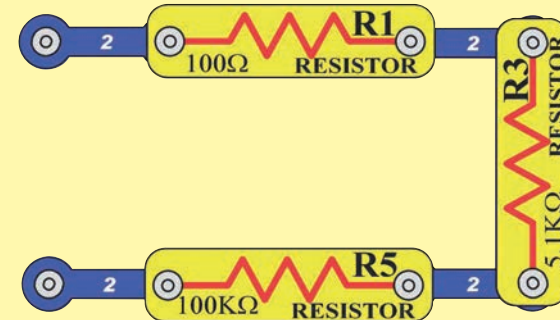
Soros Áramkör
